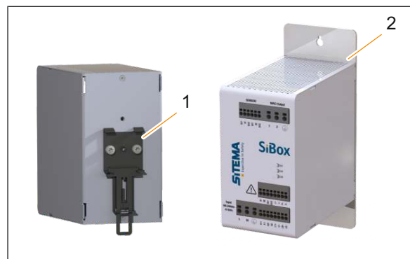
Fig. 5 : Options de montage
