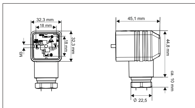
Fig. 4 : Connecteur du câble moteur
