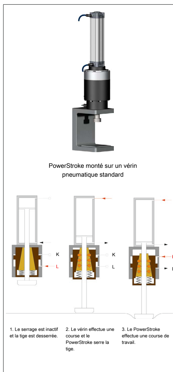
Fig. 1 : Exemple : PowerStroke FSKP sur vérin pneumatique
