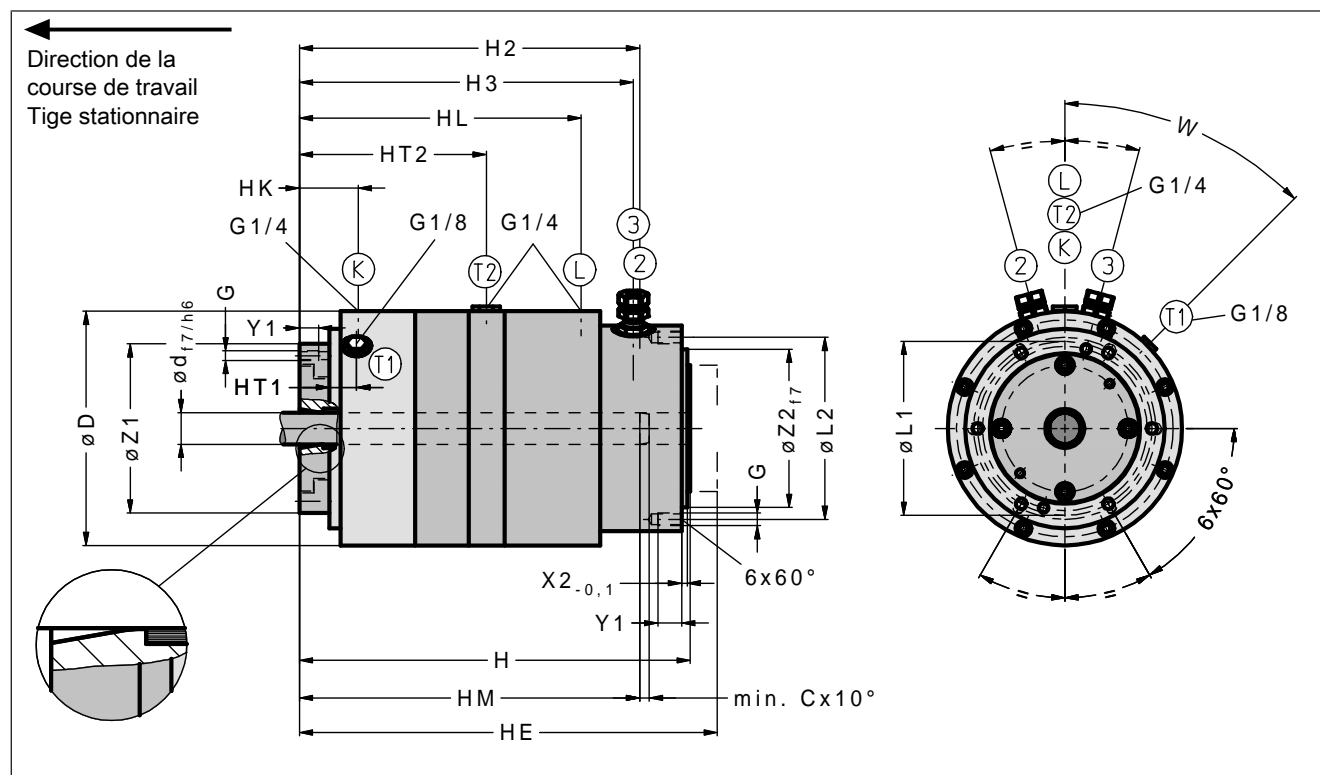
Fig. 14 : Dimensions du PowerStroke FSKP, modèle SVEL
