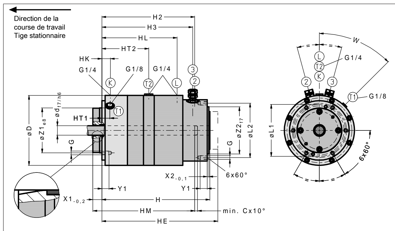
Fig. 12 : Dimensions du PowerStroke FSKP, modèle SVEF
