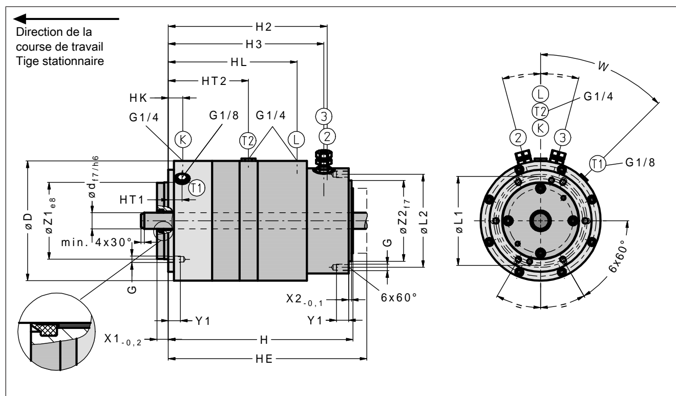
Fig. 8 : Dimensions du PowerStroke FSKP, modèle S
