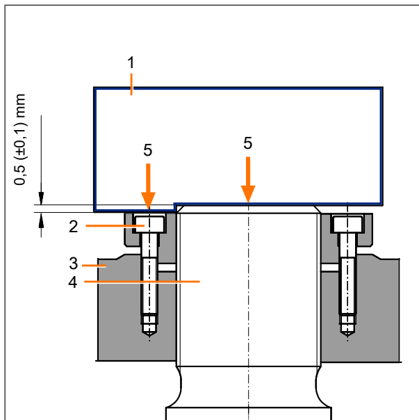
Abb. 1: Einstellhilfe, angelegt
