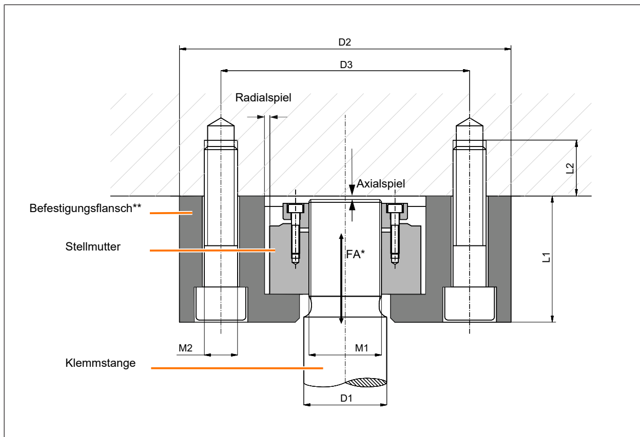
Abb. 2: Abmessungen Stangenbefestigung
