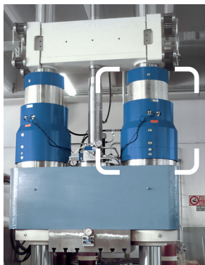
液压内高压压机 能产生 400 吨压紧力
