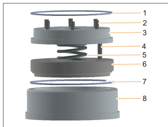
Abb. 1: Aufbau Federsockel für KSP/KSE (Beispiel)
