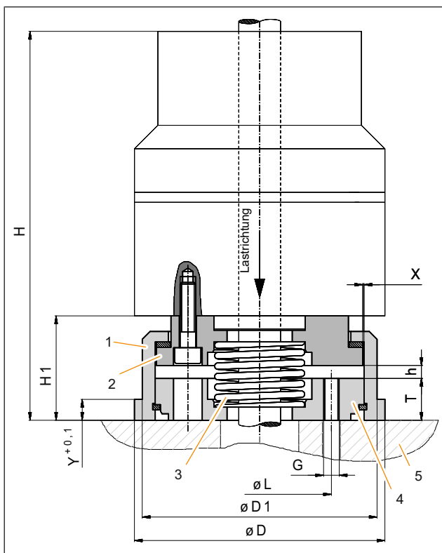
Abb. 2: Abmessungen Federsockel für Sicherheitsbremsen
