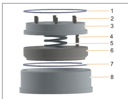
Fig. 1 : Structure de la base élastique pour KSP/KSE (exemple)
